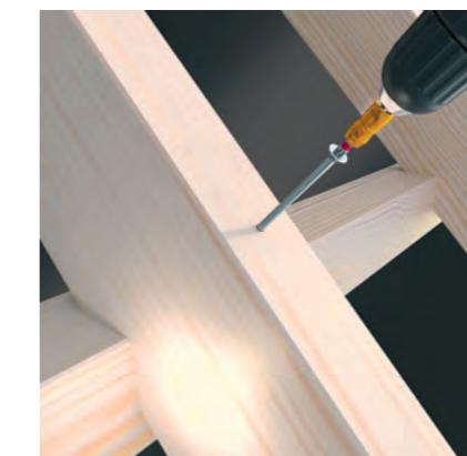
Spantbevestiging
