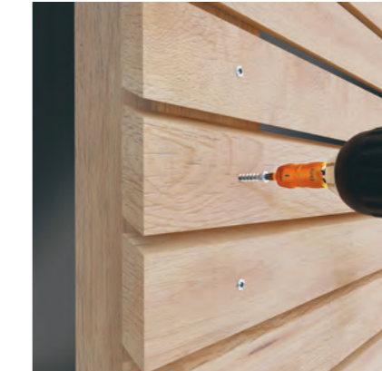
Gevelschroefverbinding
